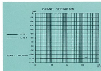
● Charakteristika Kanaltrennung
