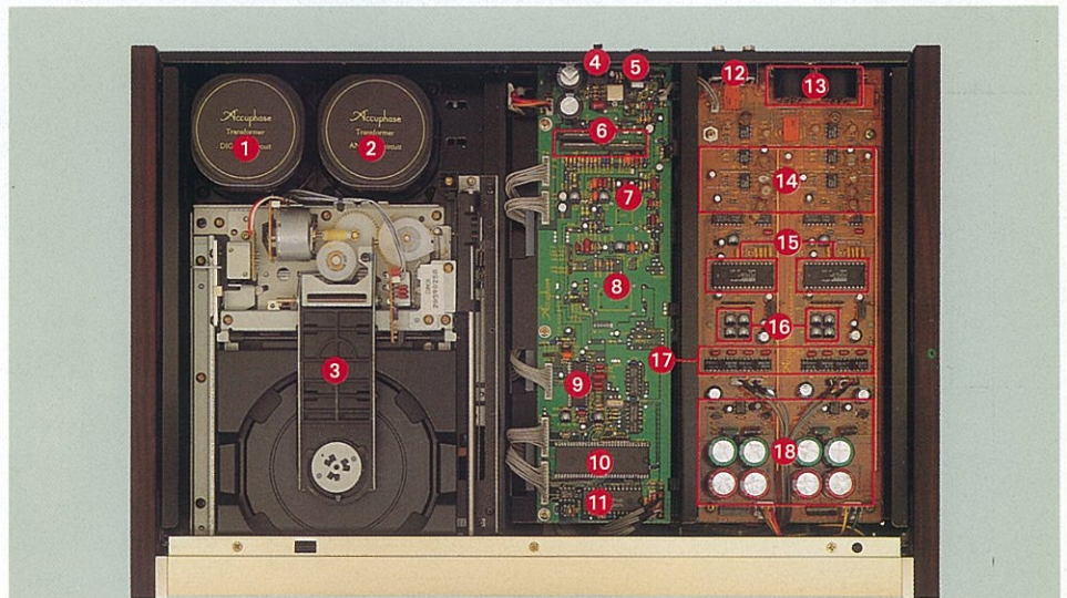
Innerer Schaltplan
