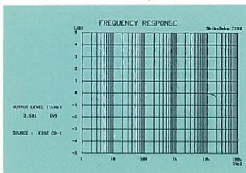
● Frequenzcharakteristika
