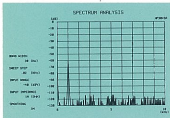
● Spektralanalyse von wiedergegebenem Signal bei 1kHz: -60 dB
