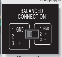
Phasenwähler
